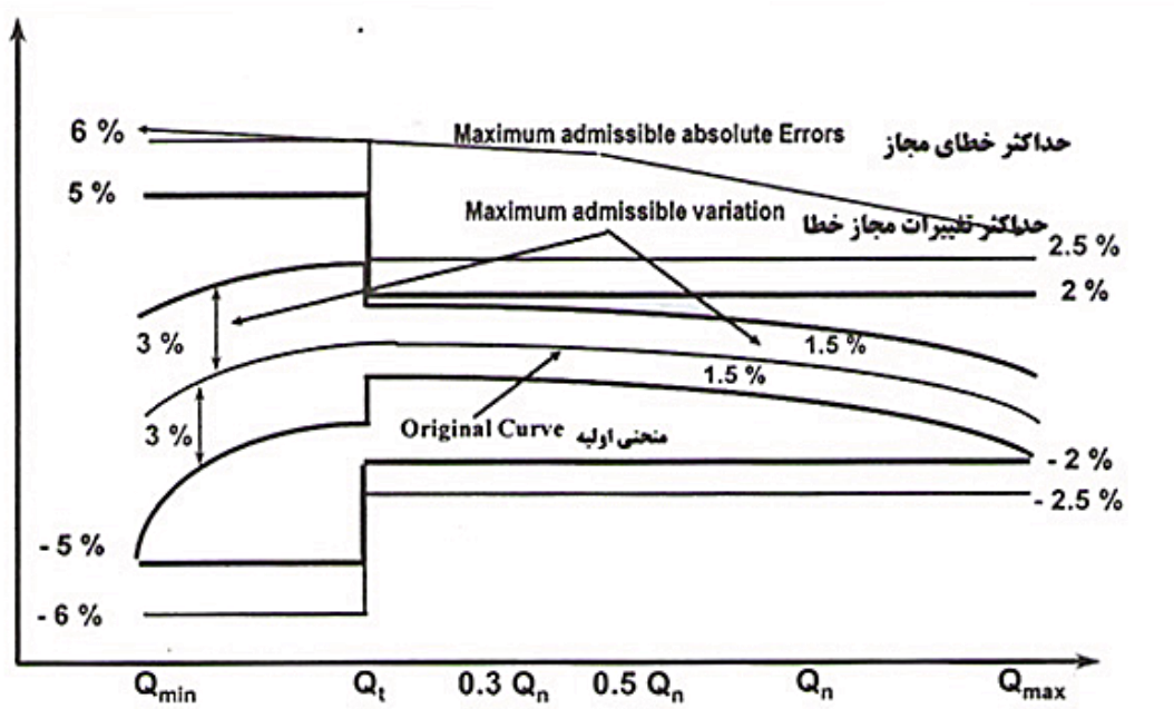
شکل ۳-۹- نمودار تقسیم بندی کنتورها و میزان خطا
