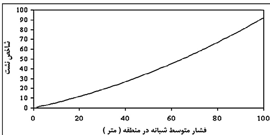
شکل ۱-۳- رابطه نشت - فشار (نشریه ۵۵۶، ۱۳۹۱)
