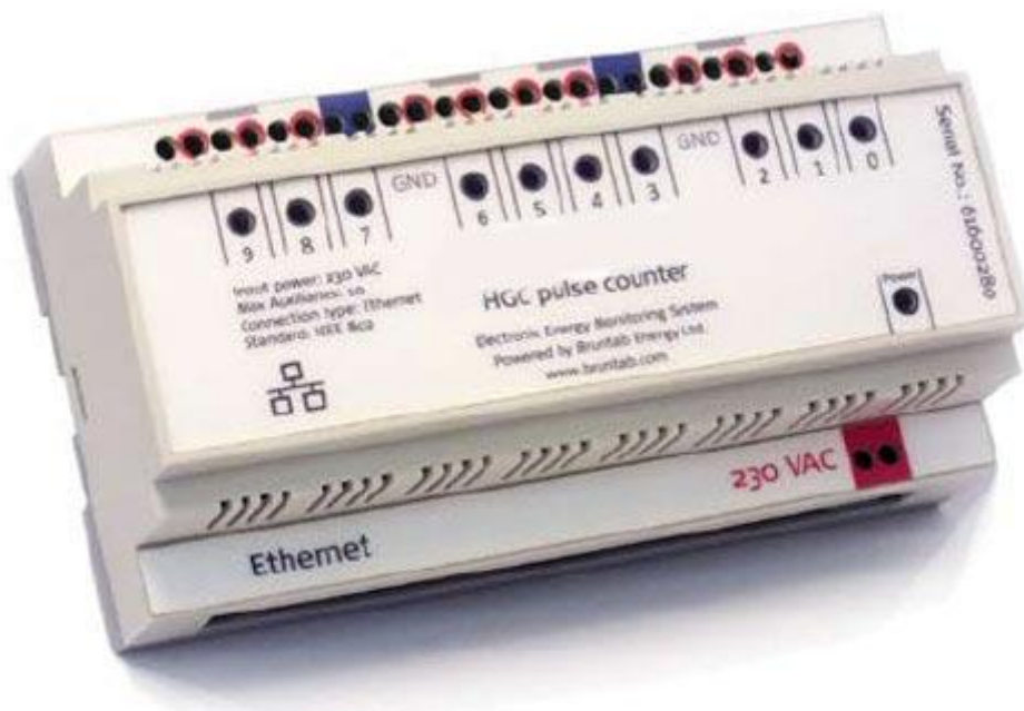
شکل ۳-۱۷- پالس شمار HGC (شمارنده پالس) در تفکیک مصرف آب
